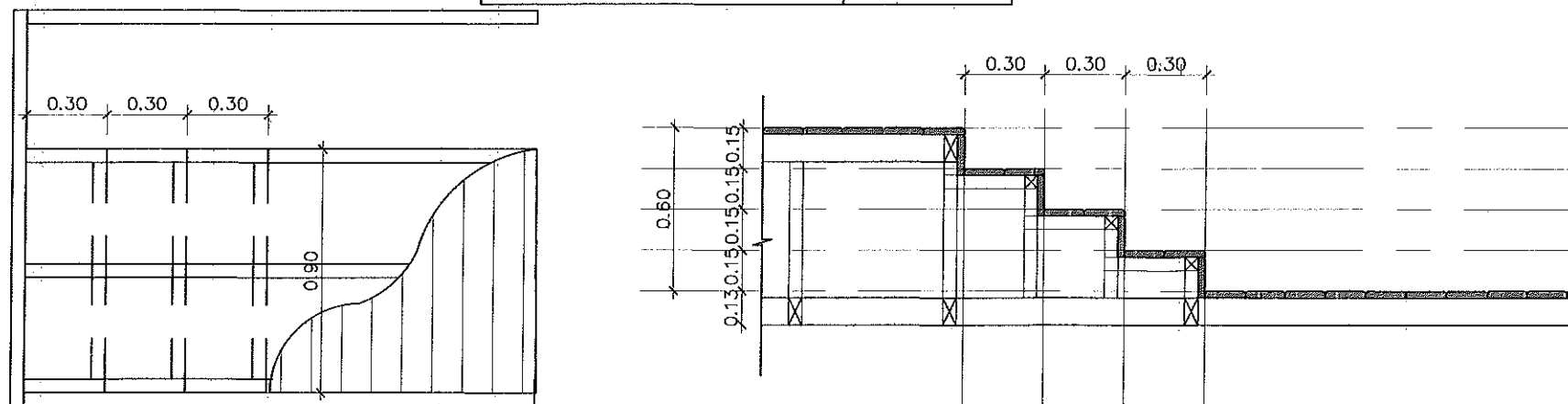
แบบขยายบ้านได้ 1 1:25
