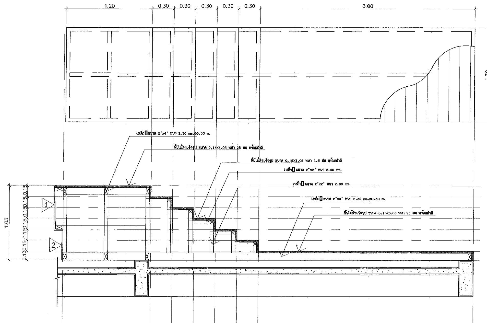
แบบขยายบ้านได้ 1 1:25
