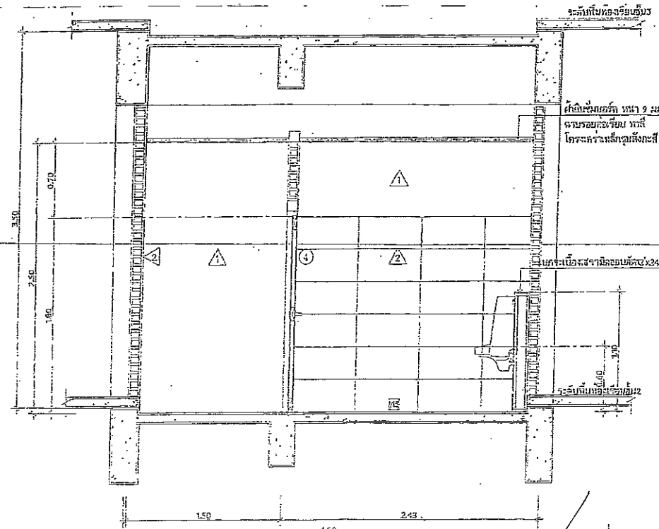
รูปตัด ③ - ③ ขนาดจริง 1:35
