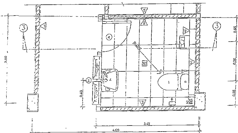
แบบขยายห้องน้ำ-ส่วน ห้องที่กด(ชั้นสอง) ขนาดจริง 1:25
