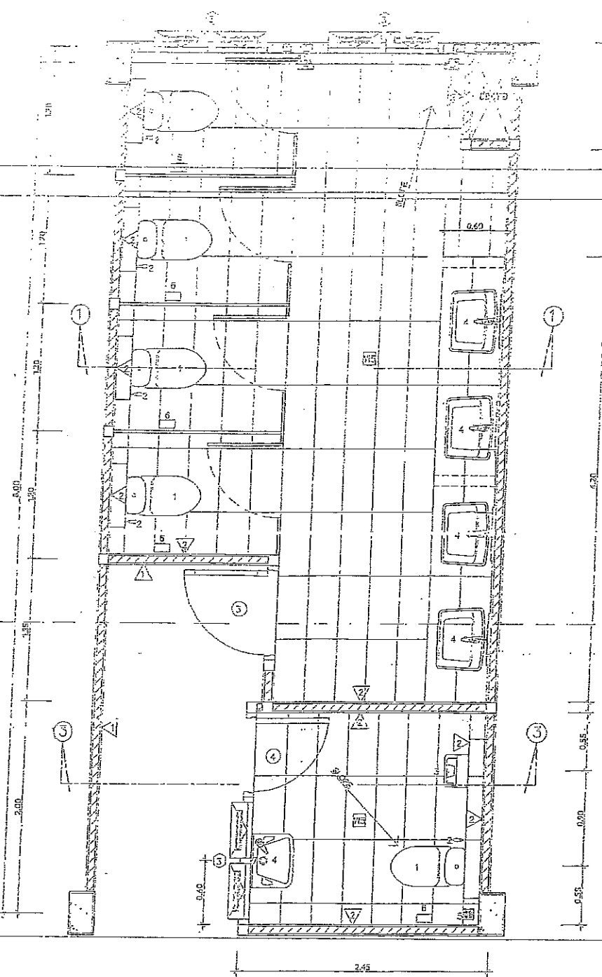
แบบขยายห้องน้ำ-ส่วน ผู้หญิง (ชั้นล่าง) ขนาด 1:25
