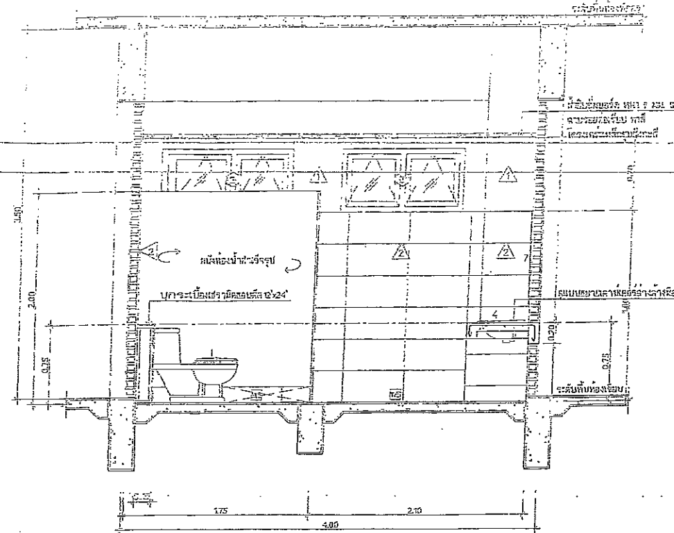
รูปตัด ① - ① ขนาดจริง 1:35
