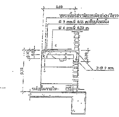
แบบขยายห้องน้ำ-ส่วน ผู้พิการ ขนาด 1:25
